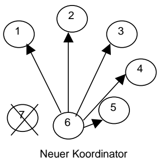
Abbildung 4-3: Arbeitsweise des Bully-Algorithmus
